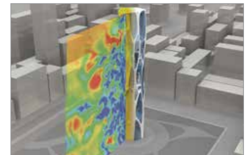
건축물의 공기 역학 해석
